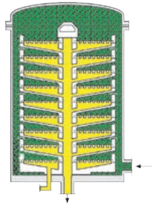
水平板式过滤器 Radium B 过滤方向：外/内
