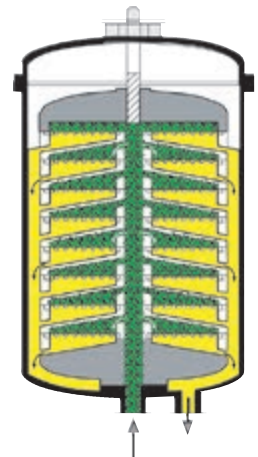
水平板式过滤器 Radium A 过滤方向：内/外
